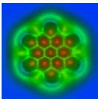
Fotografía atómica de la molécula de Pentaceno, año 2010.
